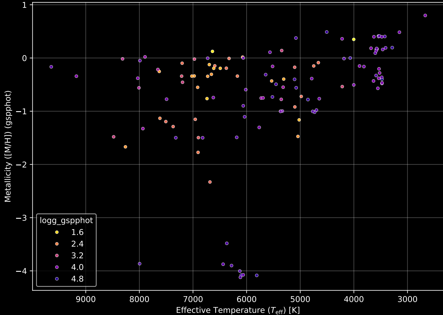
APOGEE DR17 Field: [353+17-O] Stellar Population Parameters (n= 125)
